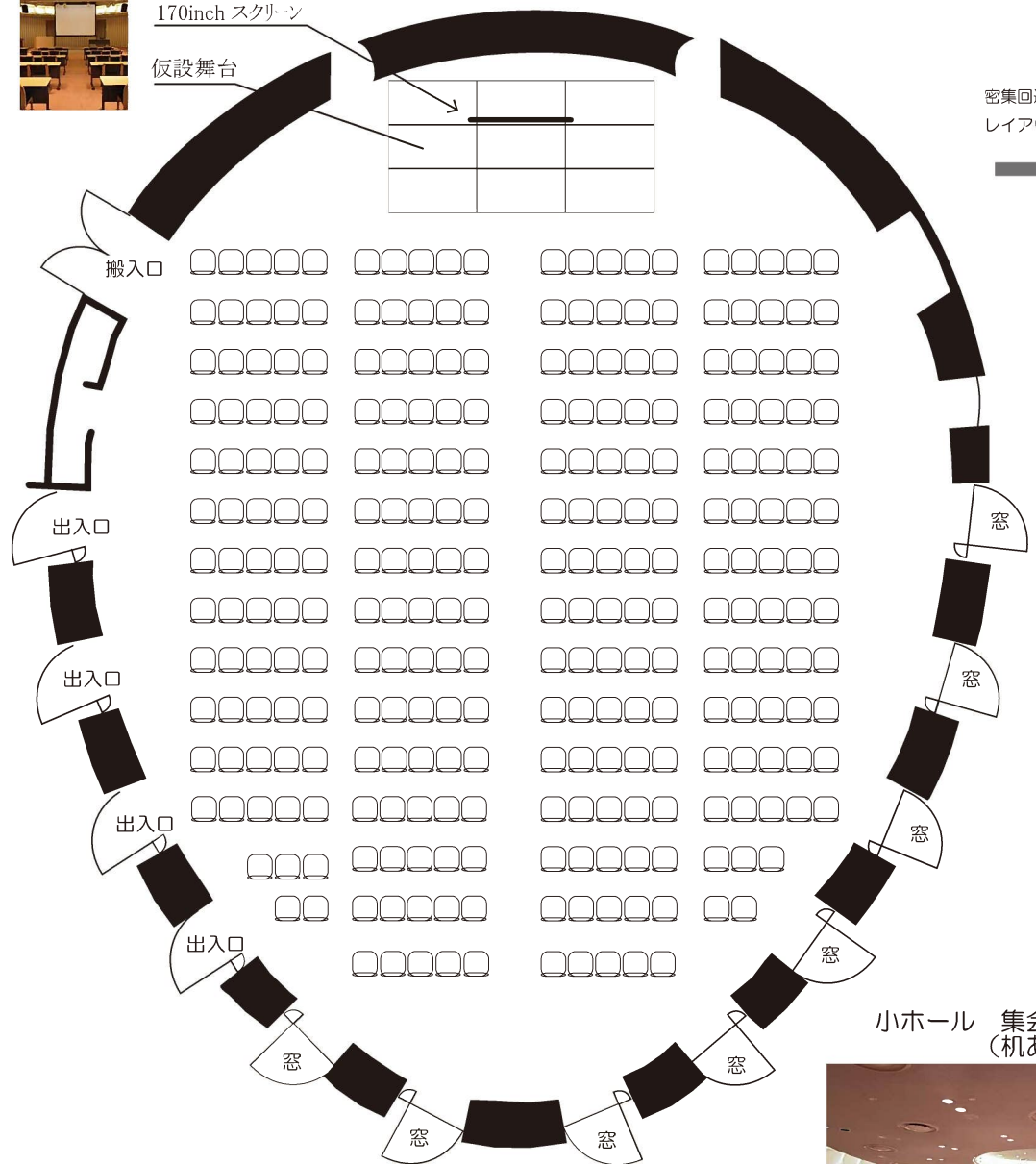
平常時 3階小ホール 集会形式平面図 280名
